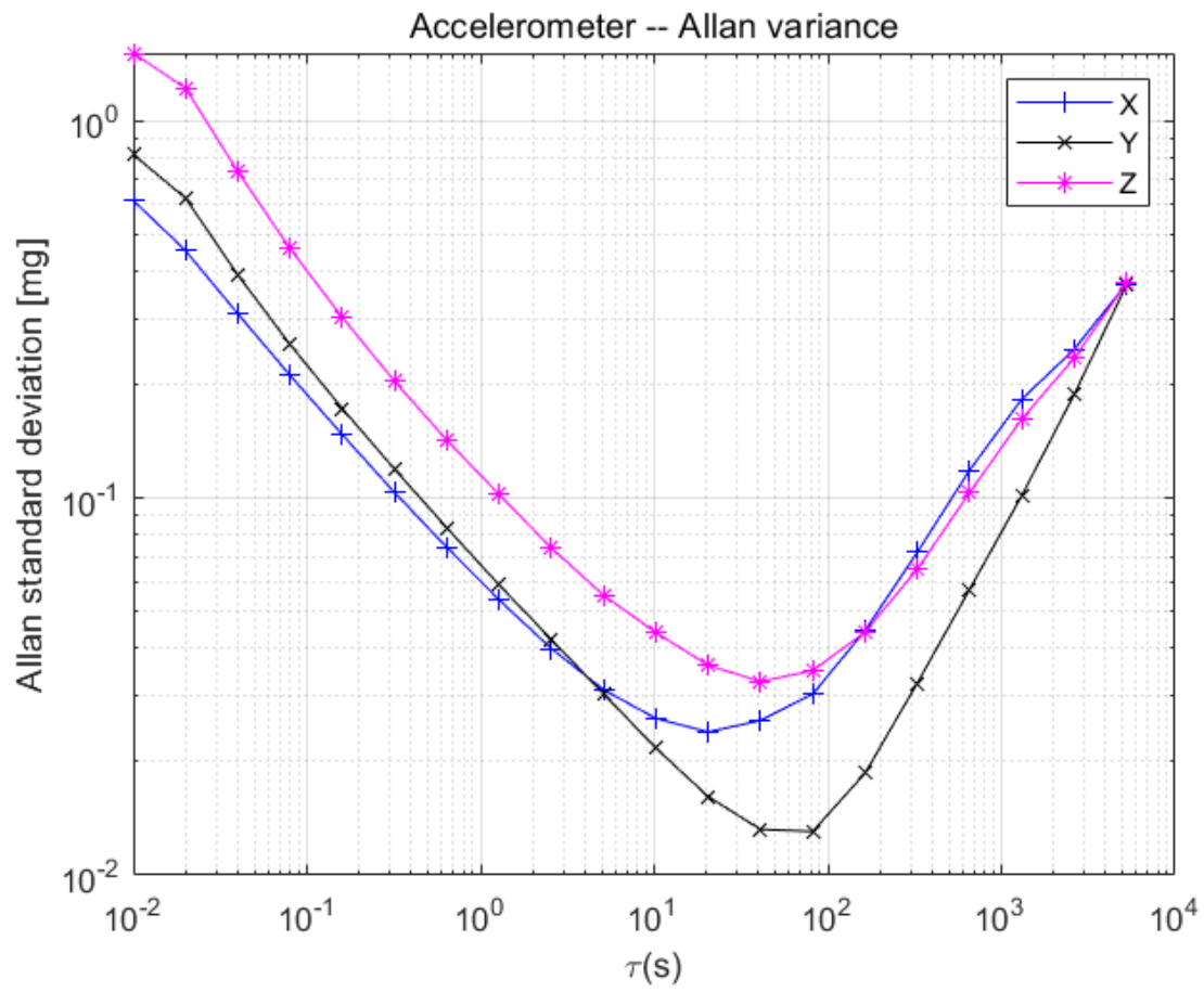
加速度Allan方差曲线(CH108)
