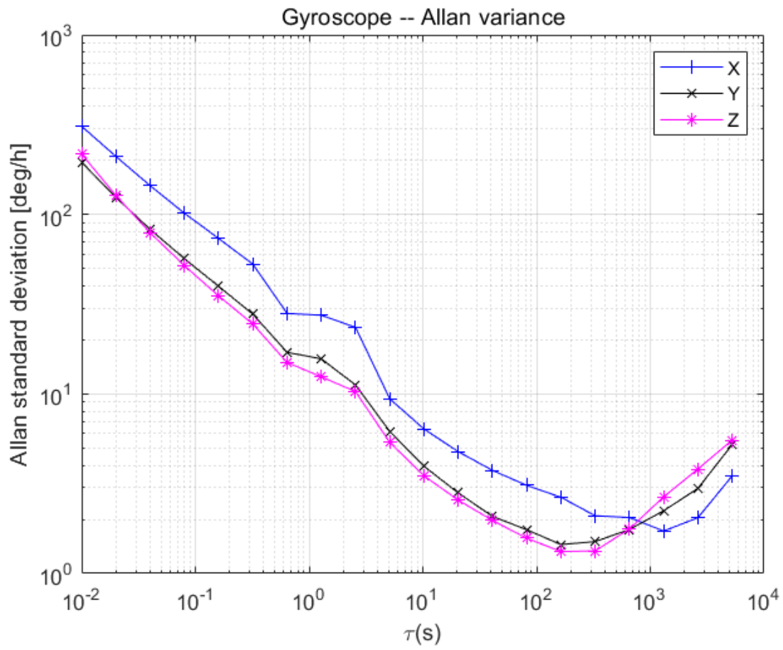
陀螺Allan方差曲线(CH108M)
