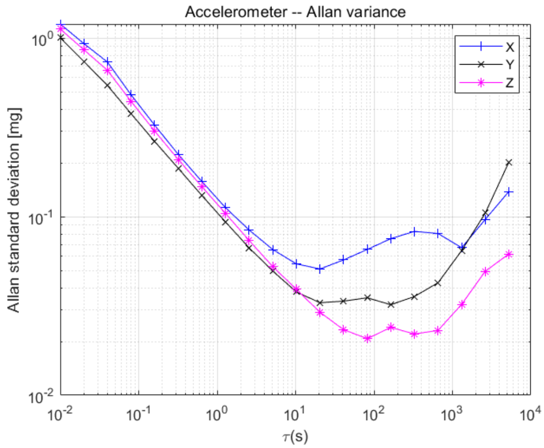
加速度Allan方差曲线(CH104)
