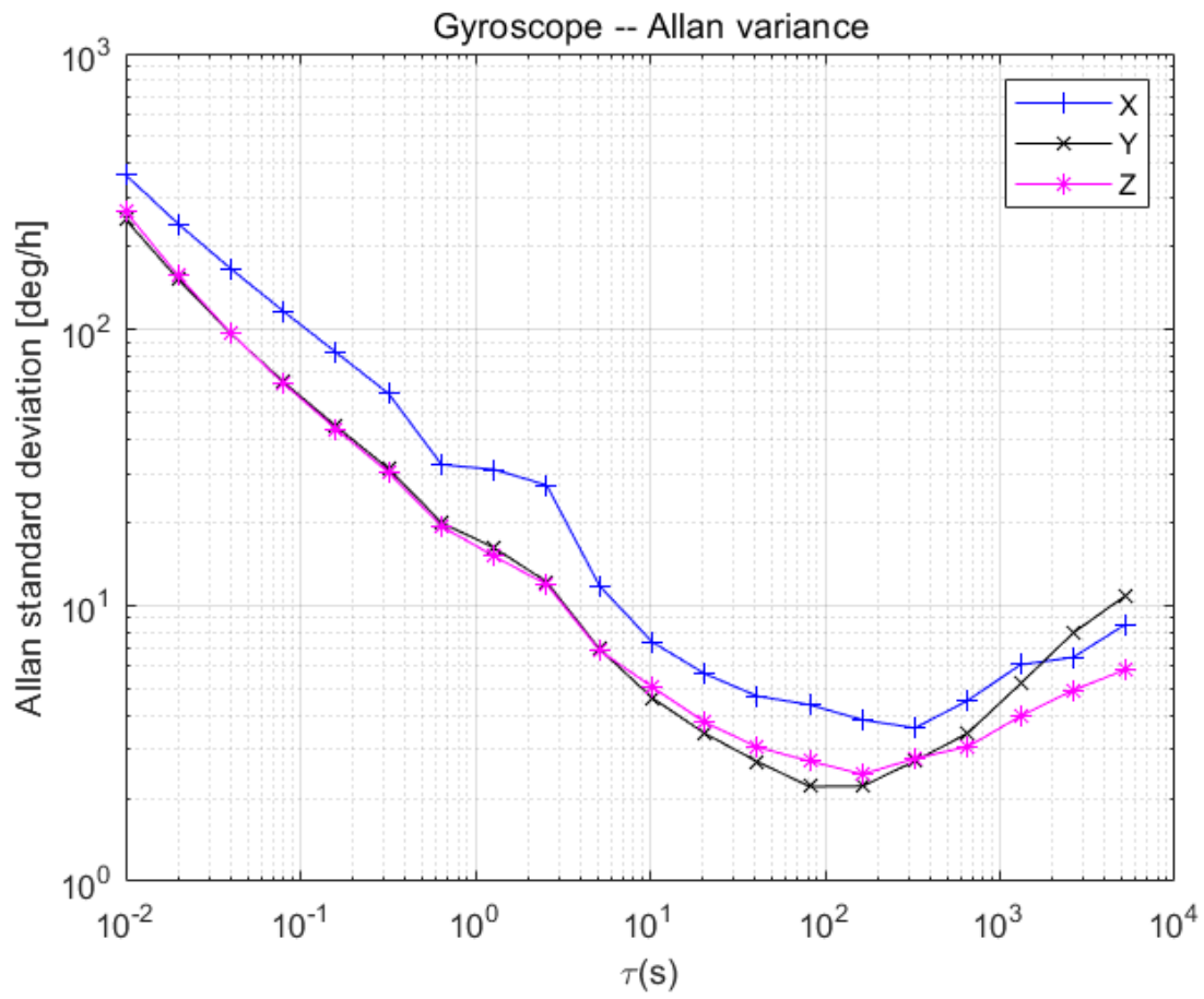
陀螺Allan方差曲线(CH104)
